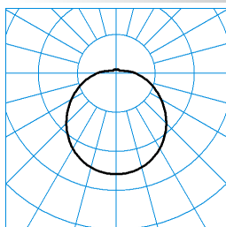
Mondia G2 WD1 LED1000-840 TX050105
